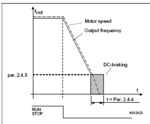
图1-12. 当“停车模式=斜坡”时的直流制动时间
