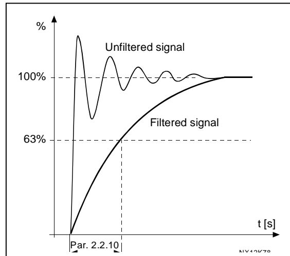
图 1-3. AI1 信号的滤波
