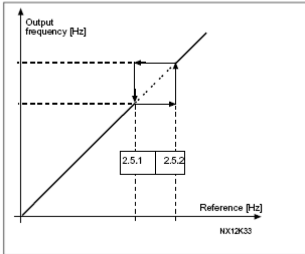
图1-14. 禁用频率区域的设置实例
