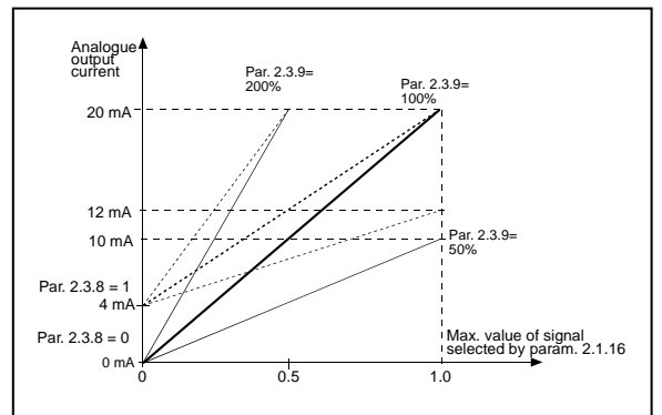
图1-7. 模拟输出定标
