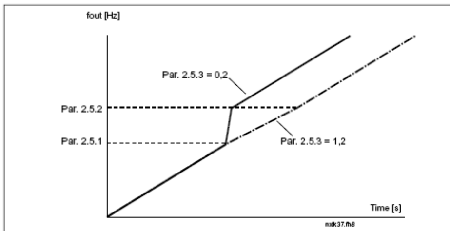
图1-15. 禁用频率加速/减速斜坡的定标
