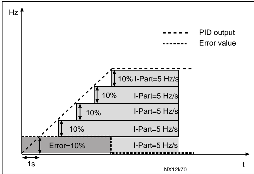
图 1-25. PID 控制器作为积分控制器的功能
