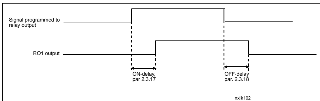
图1-1. 继电器输出1的开启和关闭延迟
