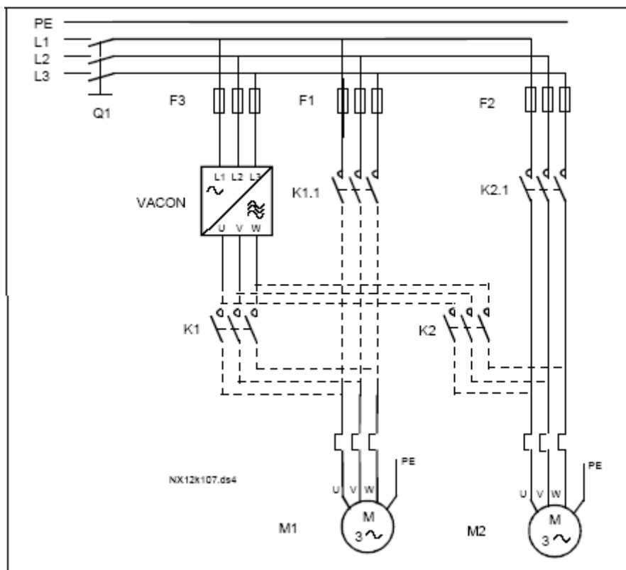
图 1-34. 2 泵自动切换主电路图
