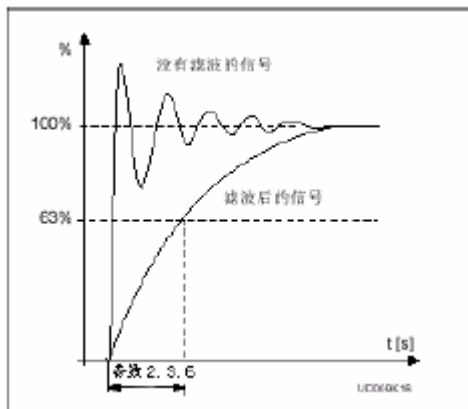
图 1-5. 模拟输出滤波
