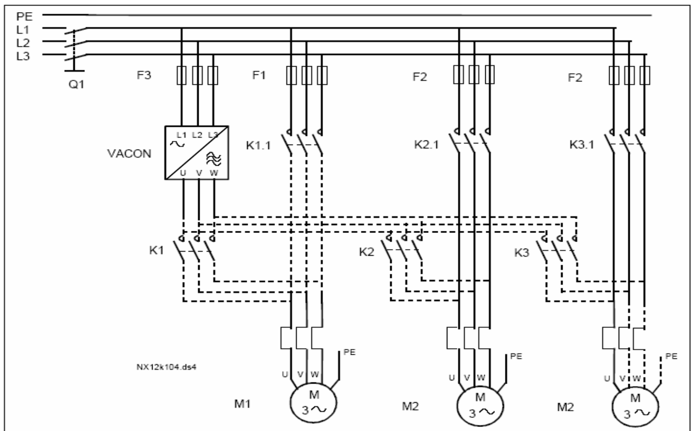
图 1-32. 3 泵自动切换主电路图
