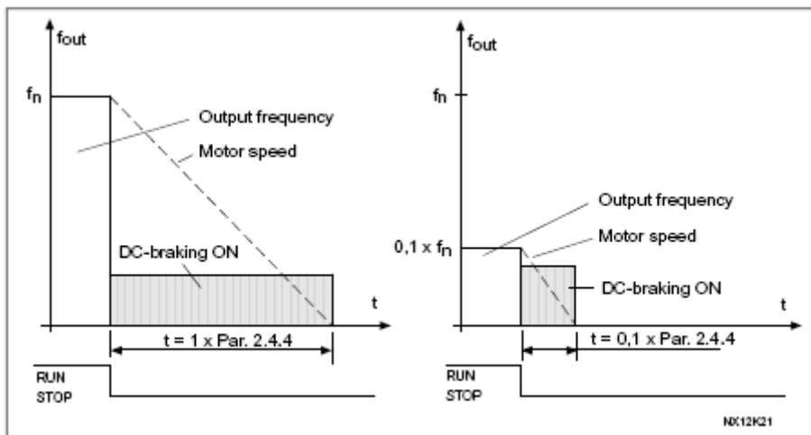
图1-11. 当“停车模式=惯性”时的直流制动时间
