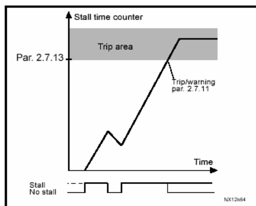
图 1-21. 失速时间计数器
