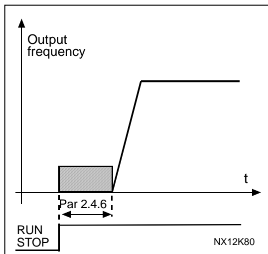
图 1-13. 起动时的直流制动时间
