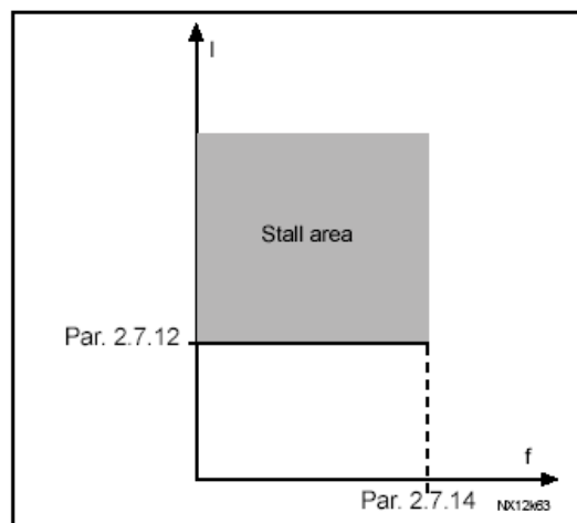
图 1-20. 失速特性设定
